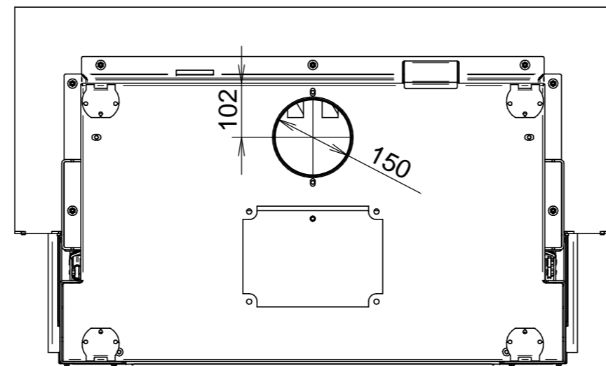
A2 / 1:10 LUNA DIAMOND DC 23 1000 GEWICHT 325KG
