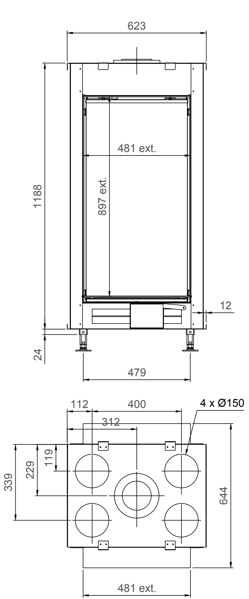
True Vision 550DV - Type 4 - 90mm
