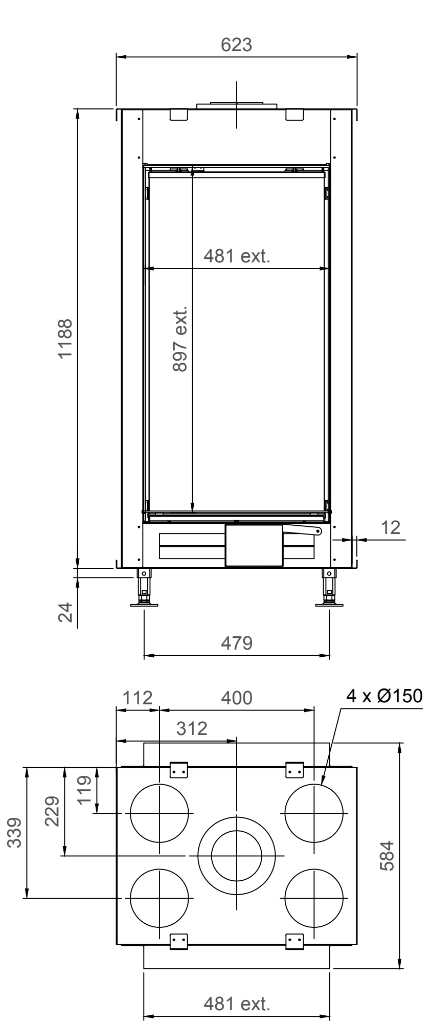
True Vision 550DV - Type 4 - 60mm
